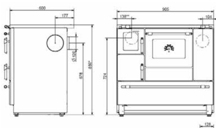
K 138CL rechts
