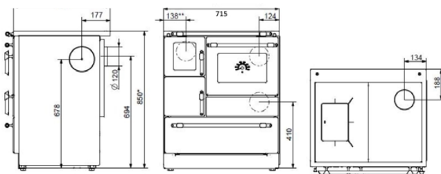
K 128CL rechts
