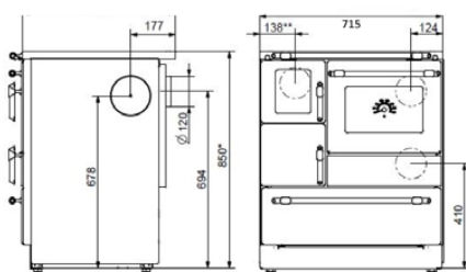
K 128F rechts
